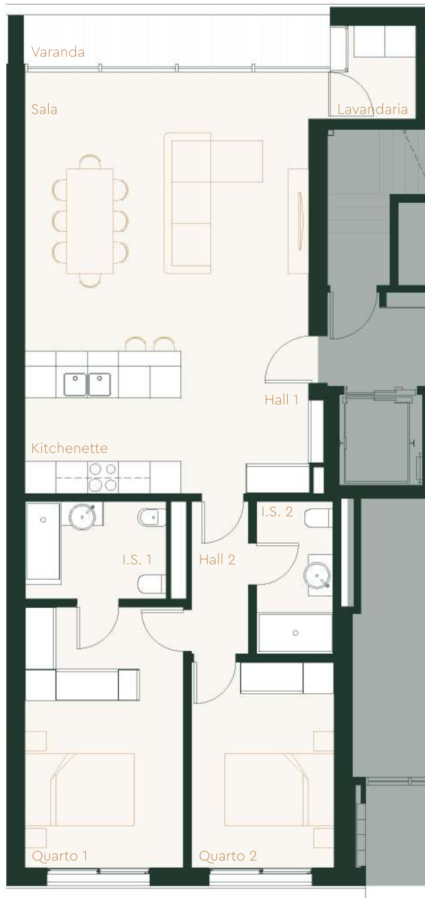
Planta da Fracção E . Escala 1:100
